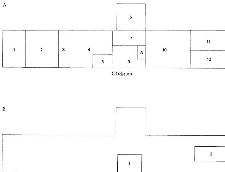
Fig 14. Vomb 1738. A visar nedre våningen, B loftet med två överflödiga kamrar, 1 och 2. A: 1 rum, 2 bryggghus, 3 spiskammare, 4 kök, 5 sängkammare, 6 överflödskammare, 7 liten kammare, 8 uppgång till loftet, 9 dagligstuga, 10 sal, 11 och 12 gästkamrar.
