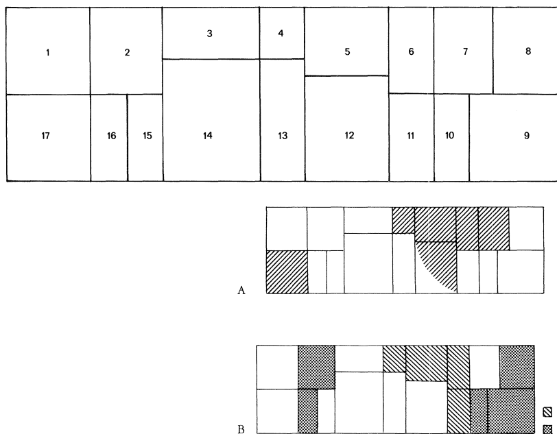
Fig 70. Högestads prästgård, byggd på 1760-talet, efter N. H. Sjöborgs beskrivning. 1 packhus, 2 morbrors kammare (även gästkammare), 3 gröna gästrummet för sämre besökare, 4 spiskammare, 5 köket med säng åt pigorna, 6 barnkammare och ammornas rum, 7 tambur (f d gamla änkefruns rum, nyttjat bl a av ambulerande hantverkare), 8 Sylwans kammare, 9 fars kammare, 10 fars farstu, 11 förmak (mors sängkammare), 12 stugan (med plats för besökande bönder och tröskarbete vid folkabordet), 13 stora förstugan, 14 salen (för släktkalas, änkekassemöten och matsal), 15 gula gästrummet (för fint främmande), 16 morbrors farstu (där barnen lekte kyrka), 17 vävkammare (här satt även skomakaren). Vid julkalasen i salen stod dörrarna till 3 o. 15 öppna. På grund av dessa uppgifter kan man urskilja samlade regioner som var avsedda till tjänstefolk, fattiga besökare och ambulerande hantverkare (A) samt manliga (2) och kvinnliga (1) regioner av bostaden (B).
