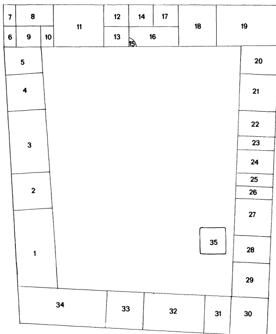
Fig 9. Gylle 1736. 1 kostall, 2 loge, 3 ladugolv, 4 högolv, 5 torvhus, 6 hemlighus, 7 kammare, 8 större gästkammare, 9 mindre gästkammare, 10 farstu med spis, 11 storstuga, 12 kammare, 13 farstu, 14 kammare, 15 källarehals(-nedgång), 16 dagligstuga, 17 kammare, 18 kök, 19 bryggghus, 20 portlider 21 drängkammare, 22 studerkammare, 23 farstu med skorsten, 24 skola, 25 svinhus, 26 hönshus, 27 portlider, 28 gåshus, 29 fårhus, 30 högolv, 31 toftaport, 32 ladugolv, 33 loge, 34 kolada, 35 gåshage.
