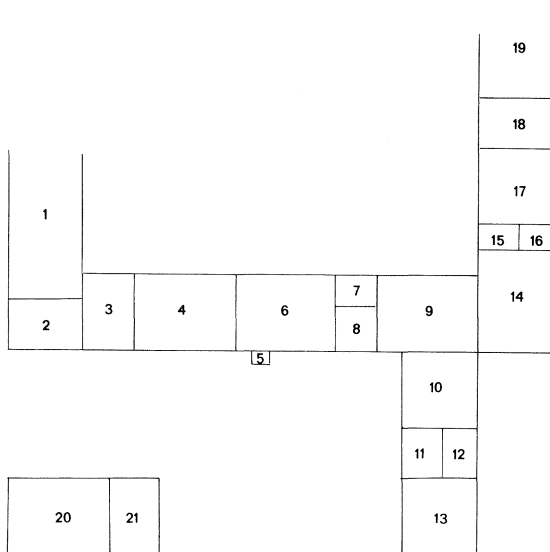
Fig 30. Billinge 1783. Boningslängan var byggd med korsvirke och lera frånsett dagligstugan, som var uppförd med bålaväggar. Köksbyggnaden skjuter ut mot gårdens baksida. 1 loge och logolv, 2 höns hus, 3 port, 4 brygghus, 5 hemlighus, 6 stuga, 7 farstu, 8 kammare, 9 stuga, 10 kök, 11 farstu, 12 kammare, 13 studerkammare, 14 sängkammare, 15 farstu, 16 kammare, 17 gästkammare, 18 visthus, 19 loge och ladugolv, 20 redskapshus, 21 torvhus. De sistnämnda båda husen hade flyttats ut efter att ha varit inrymda i en mittlänga på gårdsplanen.
