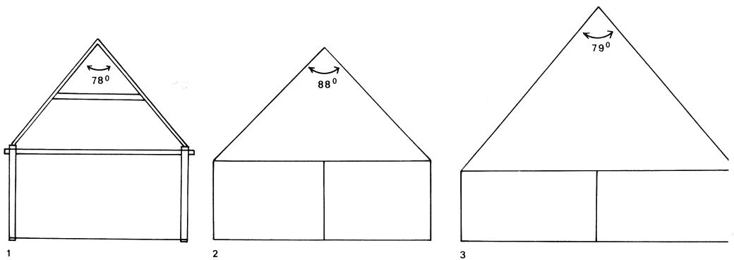
Fig 37. Bredden på bostäderna ökade. Tre tvärsektionsritningar rekonstruerade i samma skala, 1 N. Rörium 1720, 2 Bosjökloster 1802 (nybyggd), 3 V. Karaby 1827 (byggd 1815).
