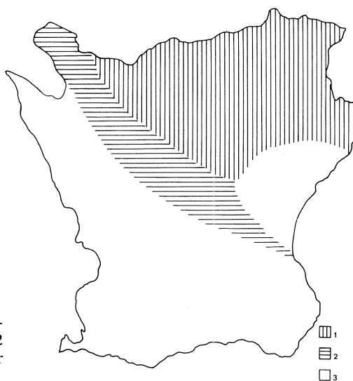
Fig 46. De olika byggnadsteknikerna i bostaden under 1700-talet. 1 knuttimring, 2 skiftesverk, 3 korsvirke. Blandtekniker förekom överallt i gränsområdena.
