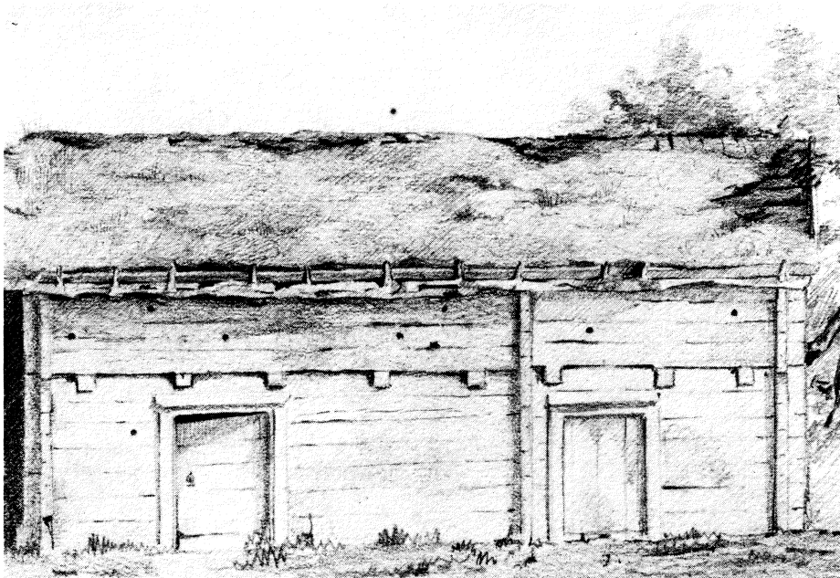
Fig 56. Knuttimrad loftbod utan någon skyddande brädpanel. Prästgården i Loshult. Teckning 1884 av R. Mejborg i Dansk folkemindesamling. Foto NM.
