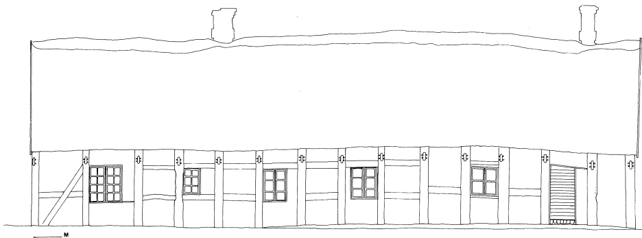
Fig 47. Den norra längan på Hjärnarps prästgård uppförd 1726 med högstolpar. LUF G 2975. Uppmätningen skedde i början av 1940-talet genom Helsingborgs museum och byggnaden finns numera i hembygdsparken i Båstad. Jfr fig 36.
