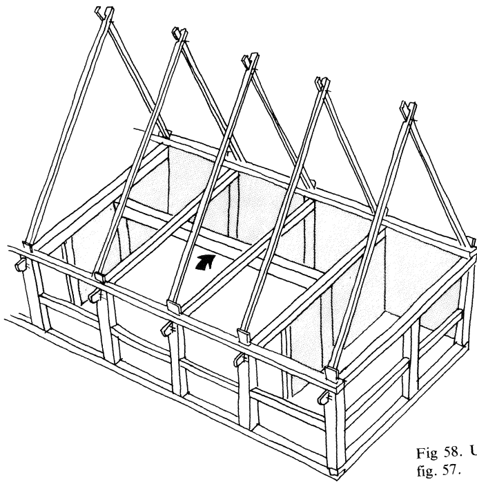
Fig 57. Ridbjälke. Principskiss efter uppgifter i synematerialet.
