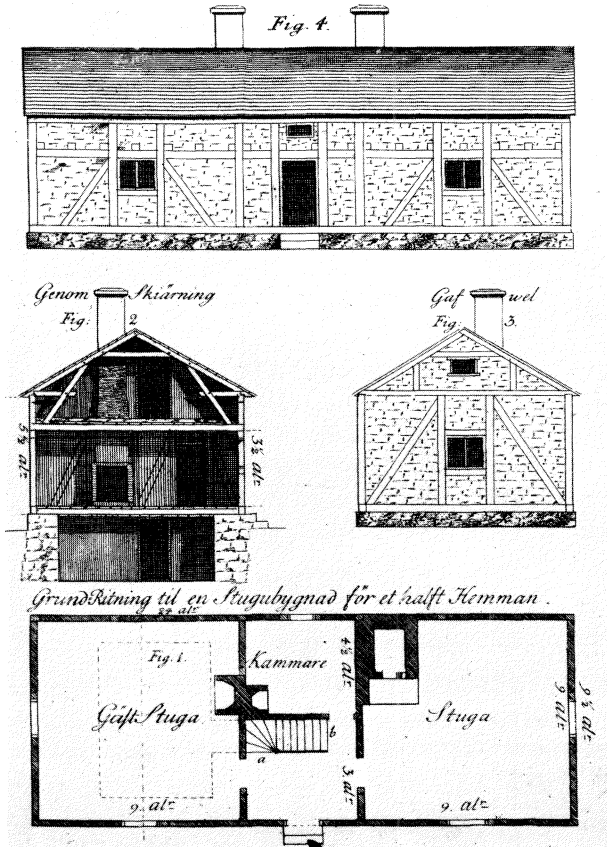
Fig 48. En manbyggnadsritning anpassad till skånska förhållanden. Wijnblad 1766.
