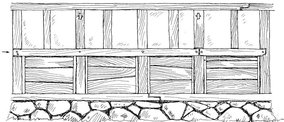
Fig 59. Listeträ. I en vägg med blandteknik, båle nederst och lera över sträcker sig ett listeträ utanpå de tre facken till vänster och ersätter löshulten. Det är infällt i väggstolparna och fastgjort med tränaglar. Ravlunda nr. 7, Albo h:d. Uppmätning av G. Gustafsson 1928 LUF G 72.
