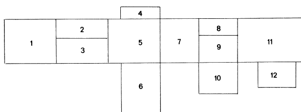
Fig 13. Tullstorp 1780. Det var mycket ovanligt att sängkammaren förlades i ett utbygge mot gårdsrummet som i detta fallet. Hela längan ansågs ”bräcklig och av ålder fördärvad”. 1 större stuga, 2 studerkammare, 3 farstu, 4 nybyggd gråstensluta till källare, 5 mindre stuga, 6 sängkammare, 7 kök, 8 spiskammare, 9 visthus, 10 bislag mot gården med två små rum, 11 bryggghus, 12 pigkammare.
