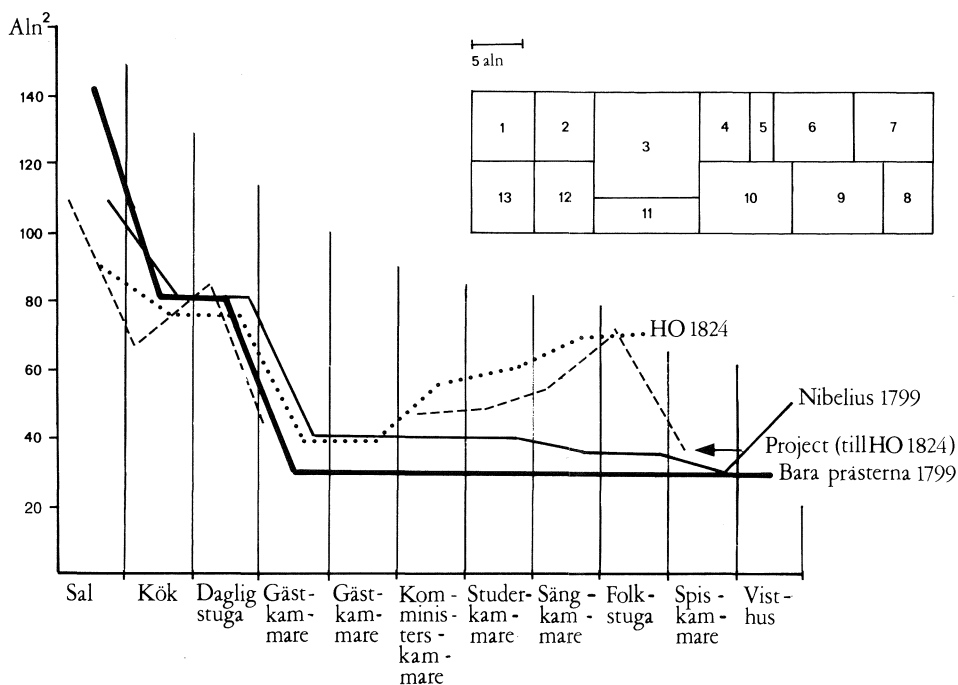
Fig 44. Prosten Nibelius i Bara kontrakt utarbetade ett eget förslag på grundval av kontraktsbrödernas synpunkter (föreg. fig.) 1 studerkammare, 2 gästkammare, 3 större stuga, 4 sängkammare, 5 klädkammare, 6 folkstuga, 7 visthus, 8 spiskammare, 9 kök, 10 dagligstuga, 11 farstu, 12 gästkammare, 13 komministerskammare.
