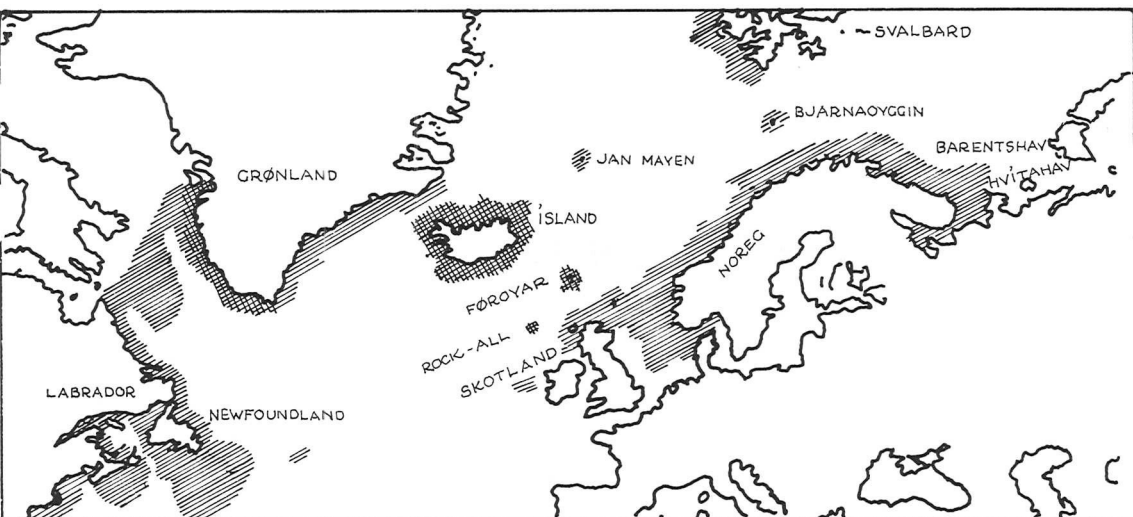
Fig. 2. Nordatlantiske fiskebanker, hvor færingerne fisker eller har fisket. Dobbelt-skraveringer viser, hvor slupperne fiskede.
