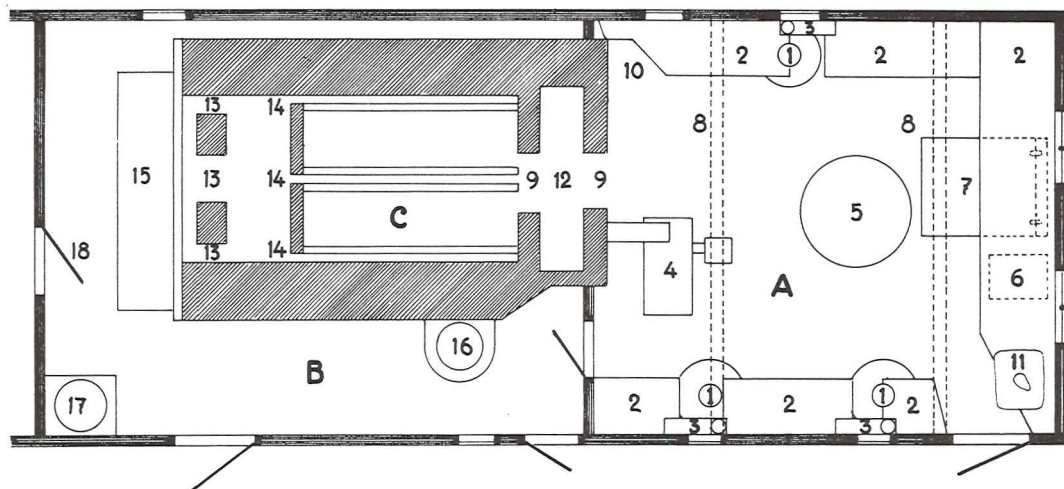
Bild 20. Plan av Törngrens krukmakareverkstad i Falkenberg på 1930-talet. A. verkstaden, B. brännskjulet, C. brännugnet. 1. drejskiva, 2. bänk, 3. slickerlåda, 4. galten, 5. en i golvet nedfälld kvarnsten där storklösen bearbetades, 6. låda under bänken där sandsten förvarades, 7. nedgång till källaren, förvaringsplatsen för leran, 8. desbom, 9. scheteln, 10. plats för teglet att mura igen scheteln med, 11. rivsten, 12. gruvan från vilken rökgången utgår, 13. eldhålen i ständarmuren, 14. schörgångarnas mynningar, 15. fördjupning i golvet där man stod, när man eldade, 16. blygrytan, 17. plats för sandstenskvarn, 18. dörr till vedboden. Foto NM.
