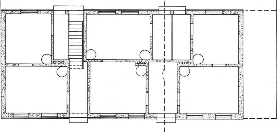
PLAN AV VÅNINGEN
